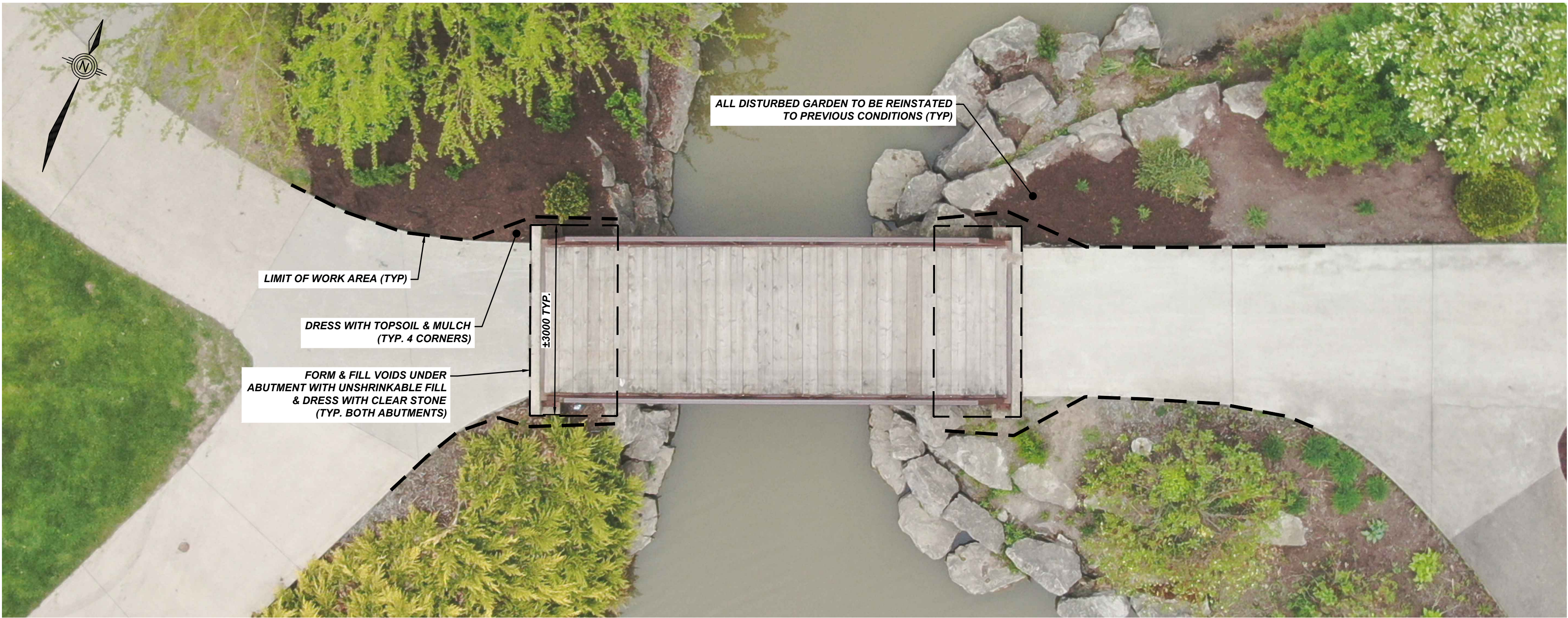
PLAN N.T.S.
