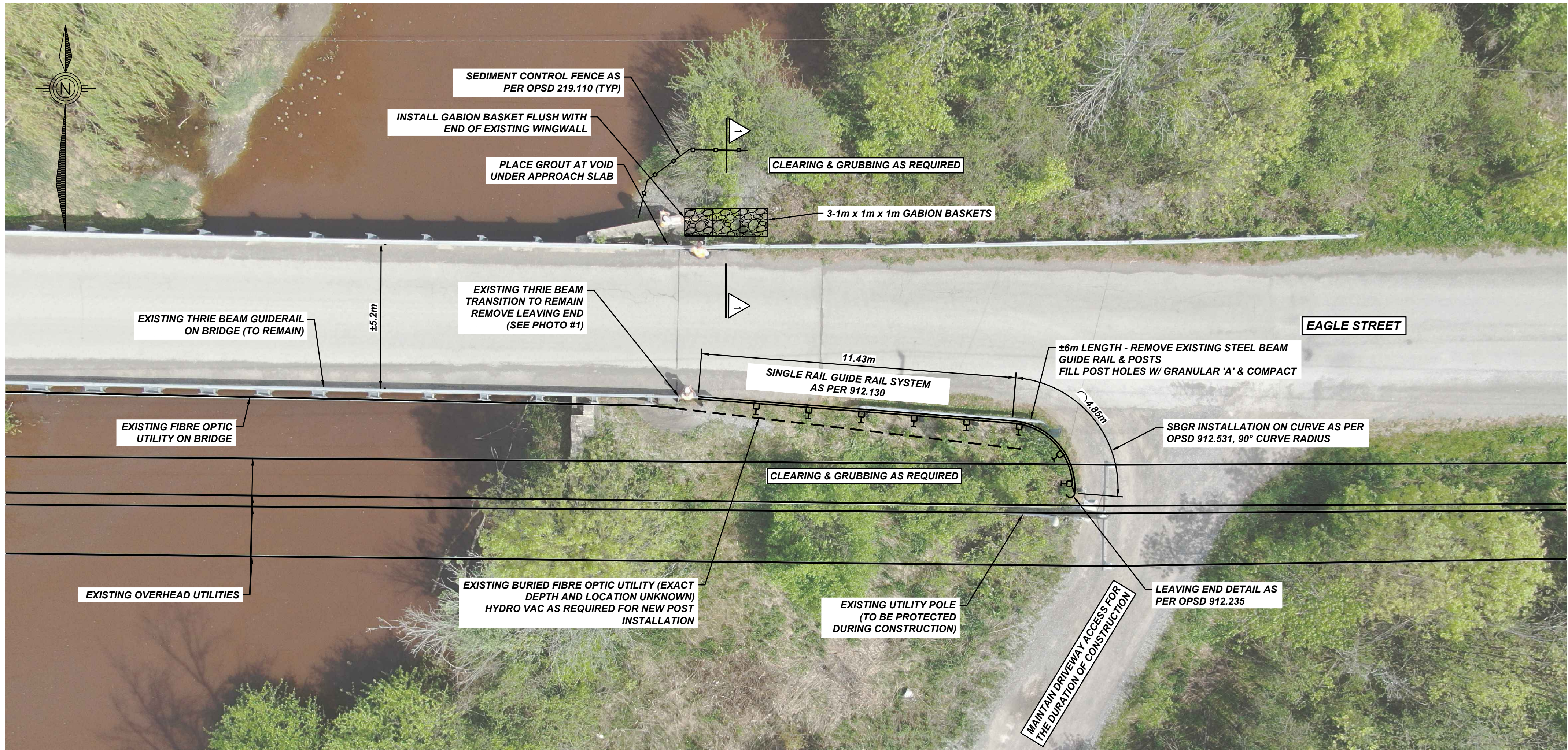
PLAN N.T.S.
